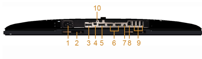
תצוגה תחתית ללא מעמד צג
